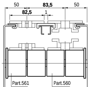
Fig. 53 - Chain width 82,5 mm (K 325) / Pitch 83,5 mm
