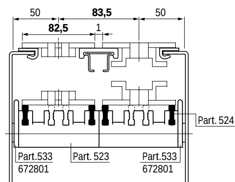
Fig. 78 - Chain width 82,5 mm (K 325) / Pitch 83,5 mm
