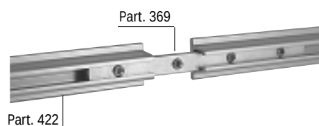
Part. 422
