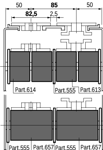
Fig. 58 - Chain width 82,5 mm (K 325) / Pitch 83,5 mm
