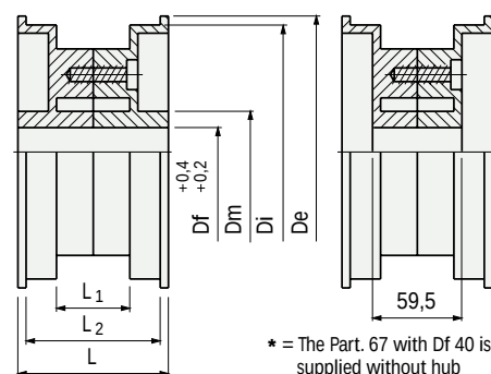
Part. 67 (Df 30) - 22 - 74
