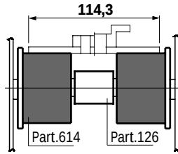
Fig. 55 - Chain width 114,3 mm (K 450)
