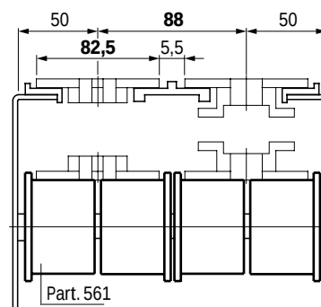
Fig. 52 - Chain width 114,3 mm (K 450) / Pitch 120 mm
