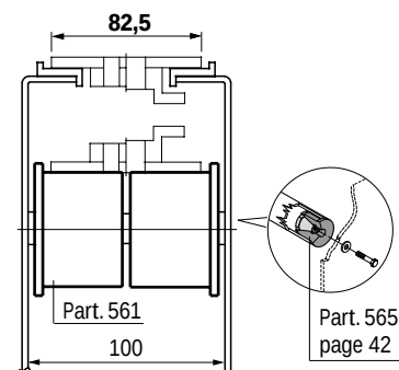
Fig. 50 - Chain width 114,3 mm (K 450)
