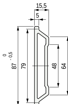
Part. 296
