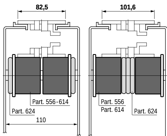
Fig. 66 - Chain width 82,5 mm (K 325); 101,6 mm (K 400)
